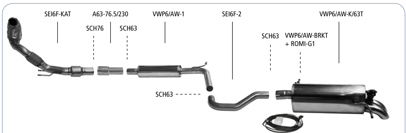
| Seat Ibiza 6F (KJ FR-Line) a partir del año 2017 | sistema de escape deportivo y catalizador de rendimiento | Silenciador trasero con válvula de escape con doble escape 2x Ø 63, 90° |
