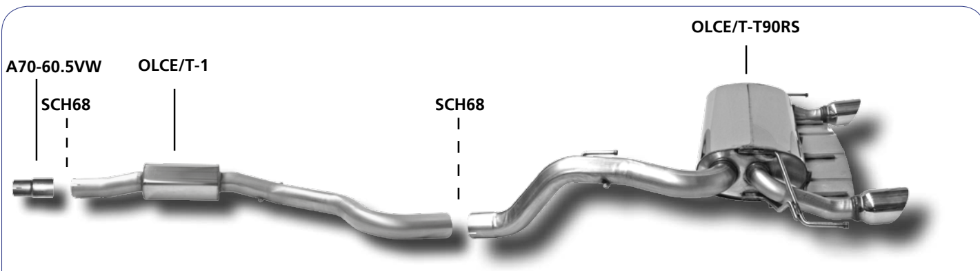
| Opel Corsa E OPC | Sistema de escape deportivo de Catalizador | Twin Silenciador trasero con 1 x Ø 90 mm RACE S tubo de salida LH+RH |
