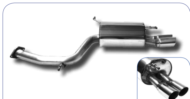
Double S | KIA SORENTO | 2x Ø 76 mm 20° | KIA/SOR-76T
